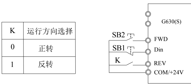
图 3-16. 三线式运转模式 2
