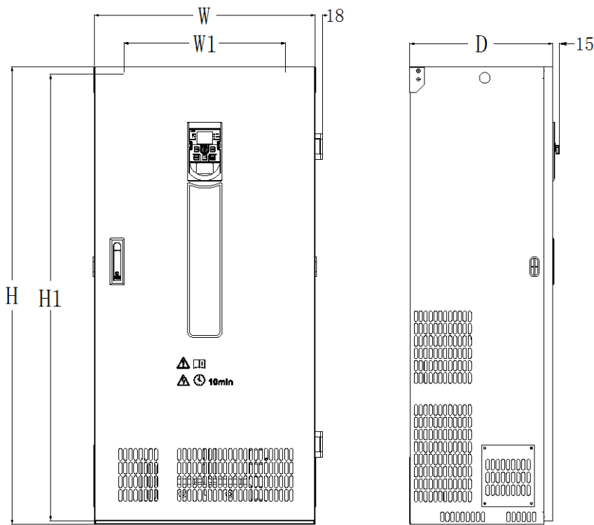
图 2-6. 380V 250kW 以上变频器外型尺寸及安装尺寸示意图
