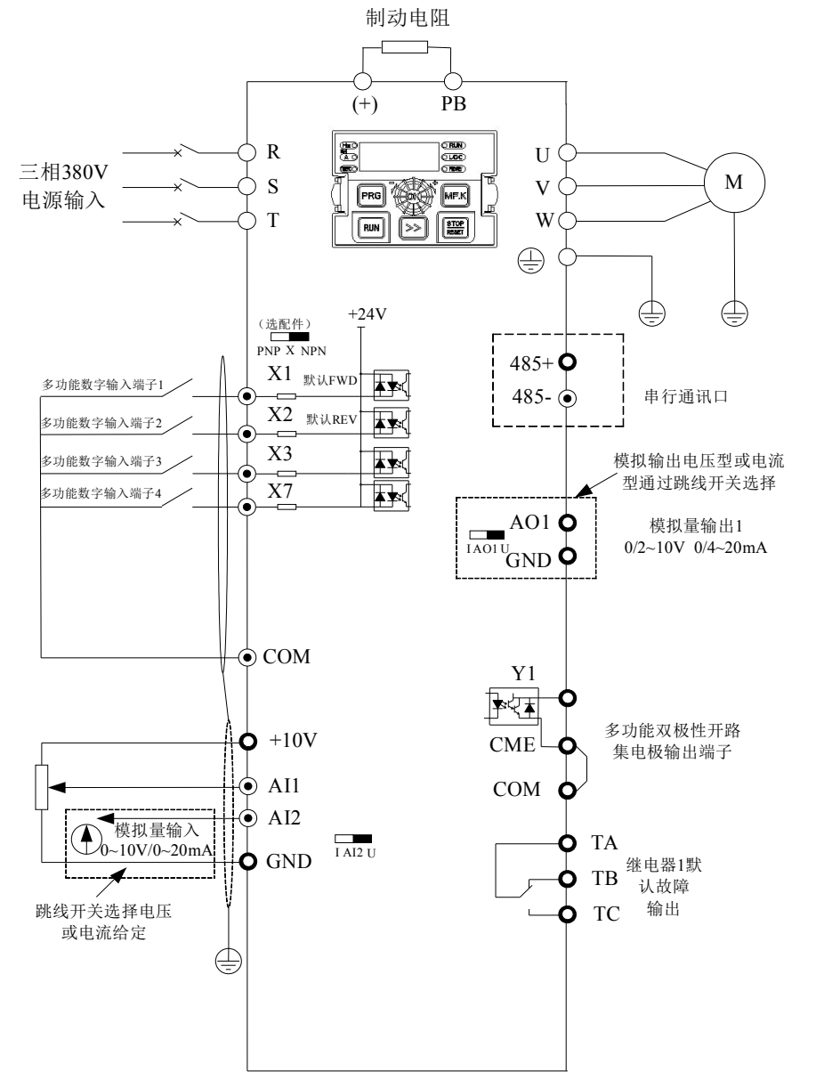
图3-1. 三相380V 2.2kW (4T:380V) 及单相220V (2S) 2.2kW(输入接L N或R T)以下变频器接线图 备注：数字输入端子X跳线开关出厂默认NPN模式（即X短接COM有效）。AI2, AO1跳线开关出厂默认电压模式。
