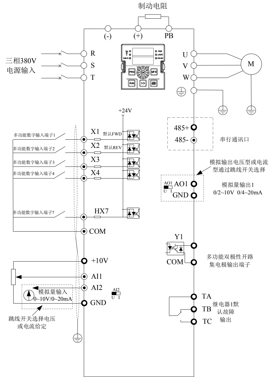
图 3-2. 三相 380V 4.0~ 37kW (4T:380V) 及单相 220V (2S) 4.0~ 5.5kW 以下(输入接 R T)变频器 接线图
