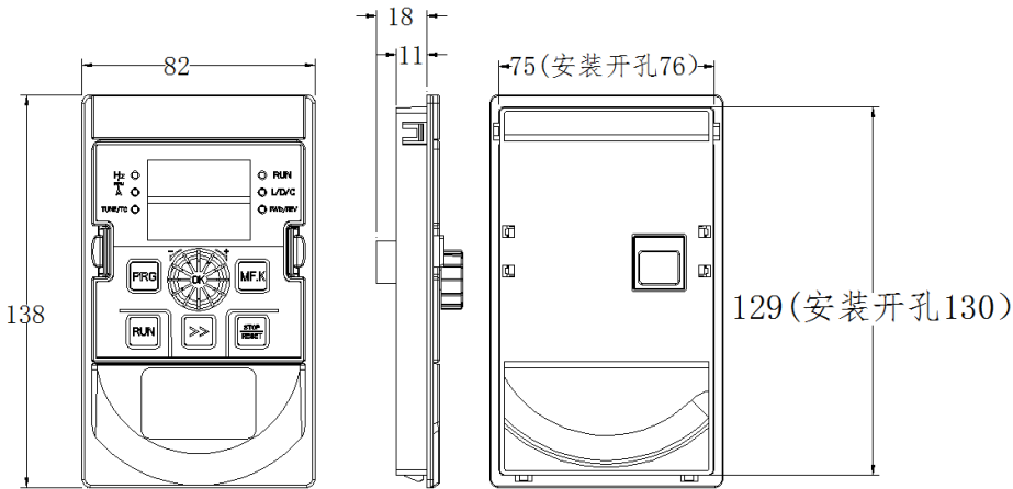
图 2-8.1 380V（4T）4.0kW以上外引键盘带托盘安装尺寸图
