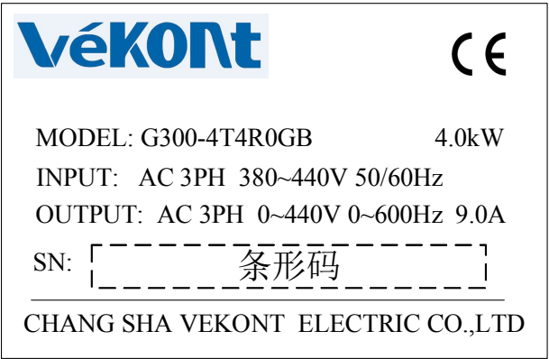
图 2-2. 铭牌
