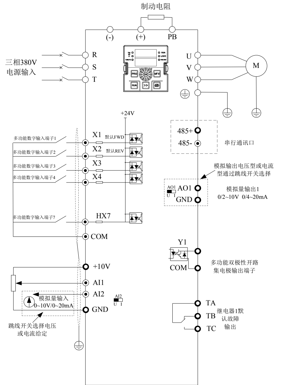
图 3-2. 三相 380V 4.0~ 37kW (4T:380V) 及单相 220V (2S) 4.0~ 5.5kW 以下(输入接 R T)变频器接线图 备注: 数字输入端子 X 出厂默认 (OP 端子连接 24V 端子) NPN 模式 (即 X 短接 COM 有效), AI2, AO1, AO2 跳线开关出厂默认电压模式。
