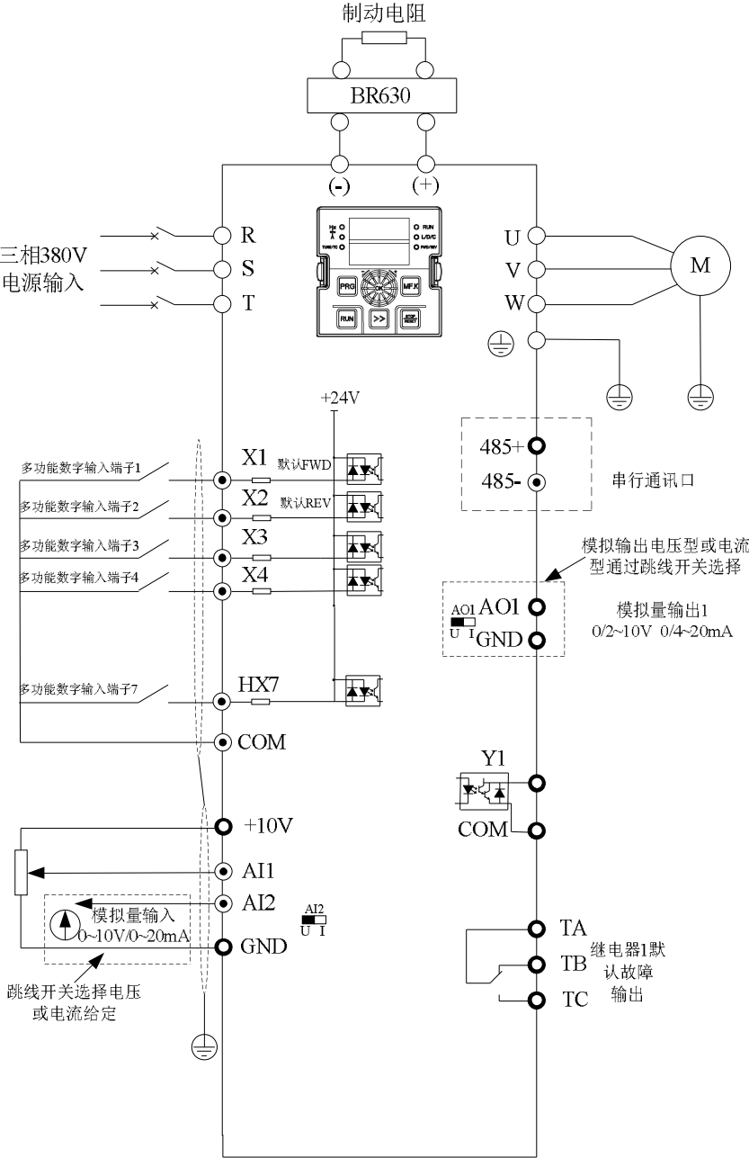
图 3-3. 三相 380V 55 ~ 110 kW (4T:380V) 变频器不带制动单元功能接线图 备注：数字输入端子 X 出厂默认（OP 端子连接 24V 端子）NPN 模式（即 X 短接 COM 有效），AI2, AO1, AO2 跳线开关出厂默认电压模式。G300/G300S 系列 37~110kW 制动单元部分属选配功能，如有需求，订货时请说明，选配了制动单元功能的接线图参考图 3-2。
