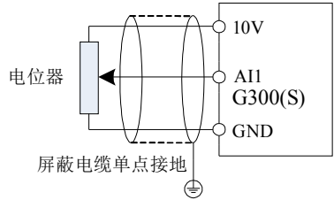
图 3-10. 模拟量输入端子接线示意图
