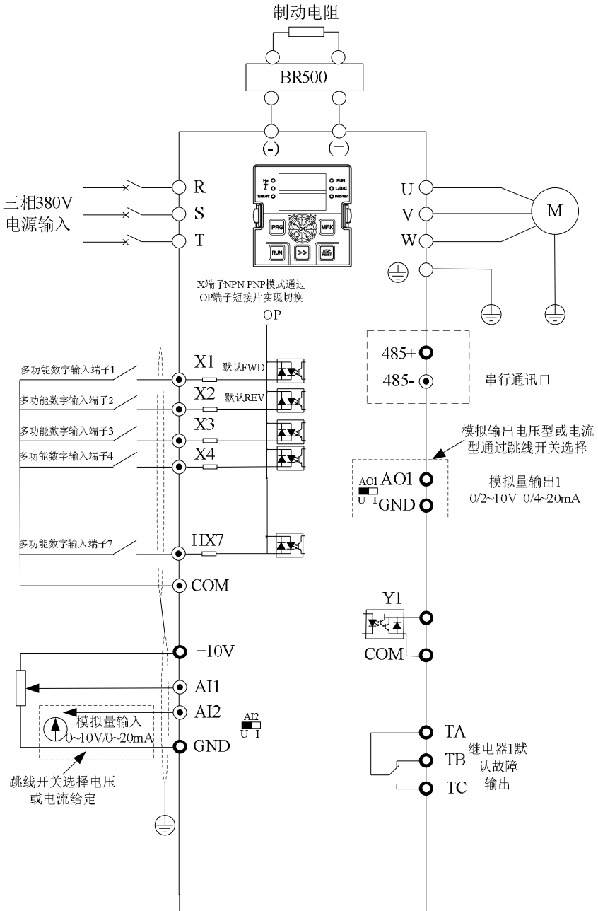
图 3-3. 三相 380V 37 ~ 75 kW (4T:380V) 变频器不带制动单元功能接线图
