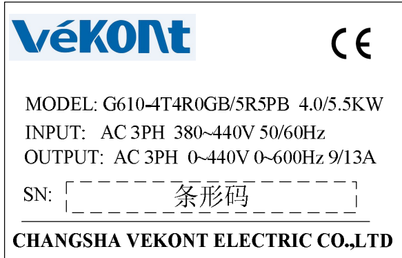
图2-2. 铭牌
