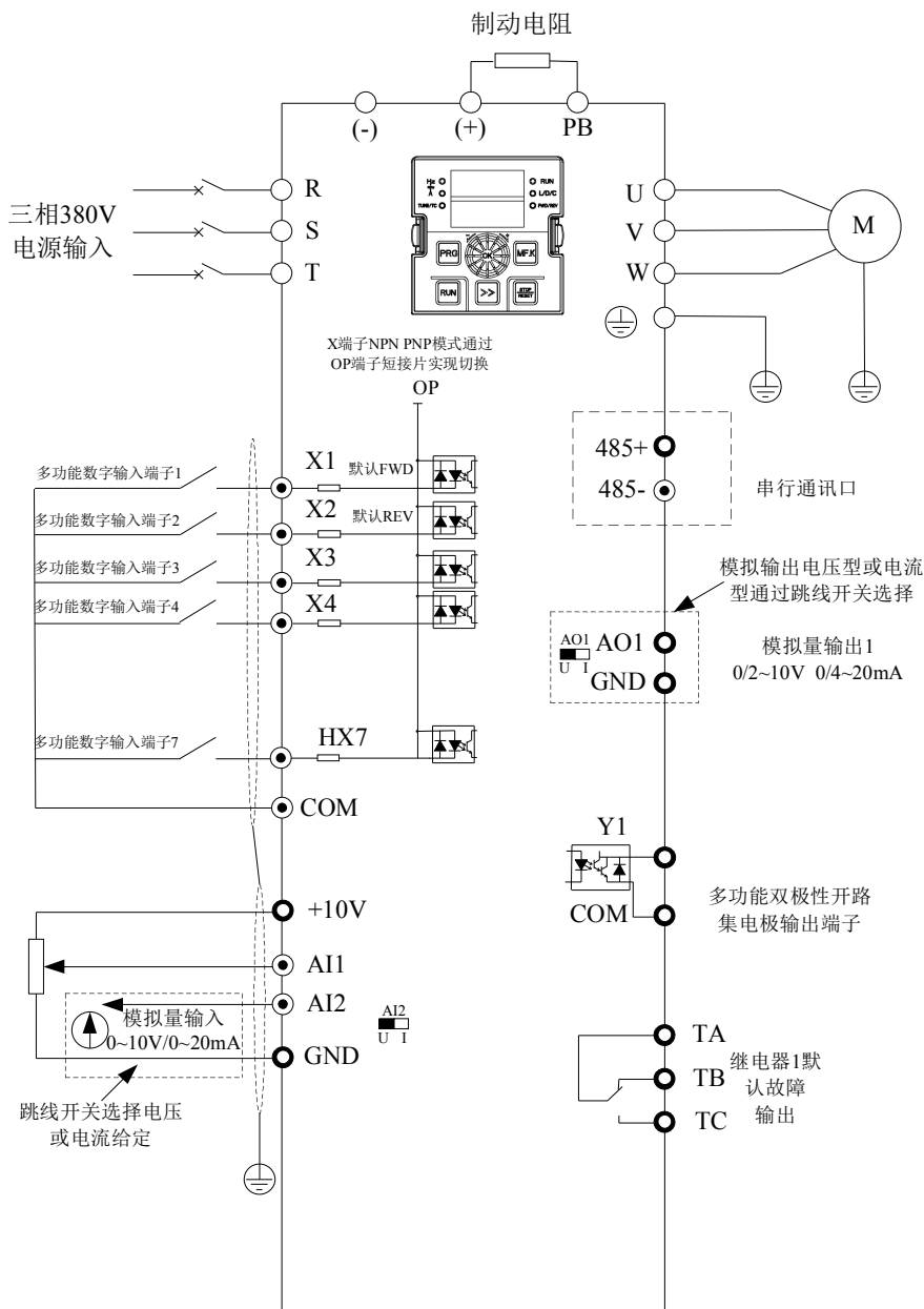
图 3-2. 三相 380V 4.0~ 30kW (4T:380V) 及单相 220V (2S) 5.5kW 以下(输入接 R T)变频器接线图 备注: 数字输入端子 X 跳线开关出厂默认 (OP 端子连接 24V 端子) NPN 模式 (即 X 短接 COM 有效), AI2, AO1, AO2 跳线开关出厂默认电压模式。
