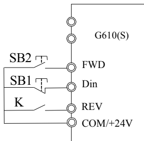
图 3-16. 三线式运转模式 2
